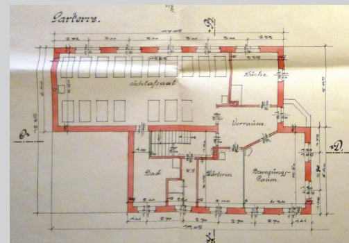
Stavební plán přízemí a prvního patra budovy dětského domova na hřišti Českého srdce v X. okrese.
